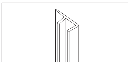
Guarnizione gocciolatoio verticale. Vertical drip seal cod. RIC107
