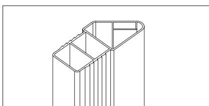
Guarnizione calamitata di battuta. Closing magnetic seal cod. RIC141
