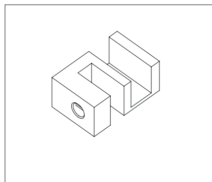
Guida di scorrimento destro. Right sliding guide. RIC136
